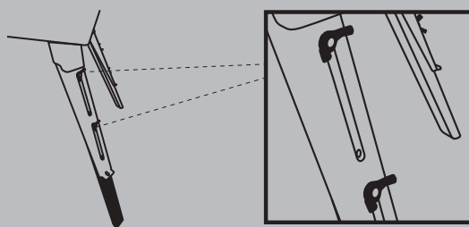
脚1本に対して2本の蝶ボルトで固定する
