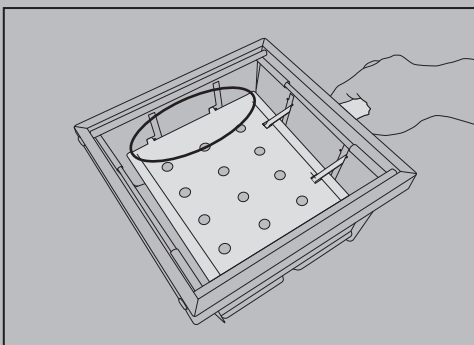
3-2. リフターを使ってロストルをスライドさせ、お好みの高さの溝に、ロストルの4カ所のツメをはめ込みロックします。
